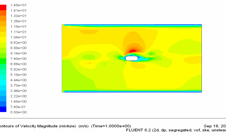
شکل 4- به ترتیب از بالا: کانتورهای فشارمطلق، فشار دینامیکی و سرعت
