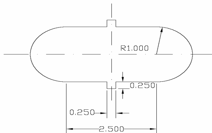
شکل 1- ابعاد هندسی بویه مورد بررسی
